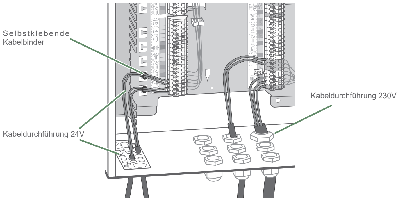
Abb.8 - Zugang zu den Klemmen
