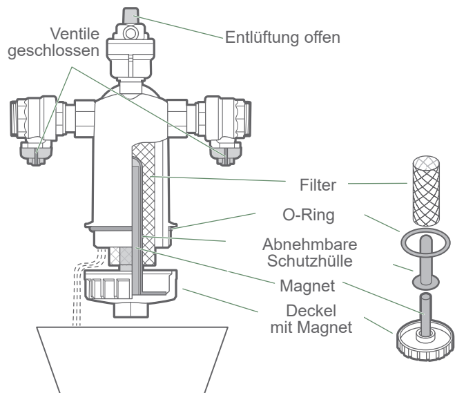
Abb.13 - Reinigung des Schlammtopfs
